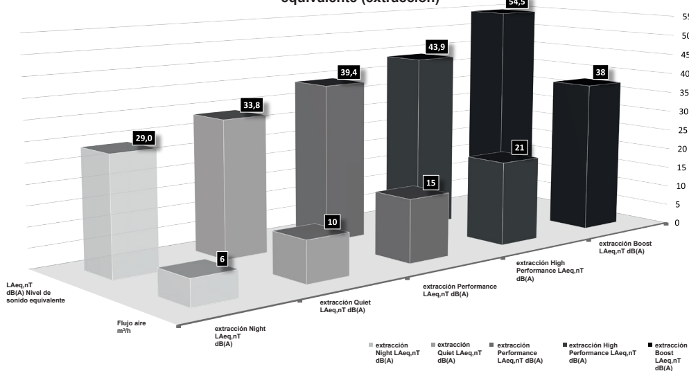
VORT HRW 30 MONO EVO WiFi - Gráfico Flujo aire / Nivel de presión de sonido continuo equivalente (extracción)
